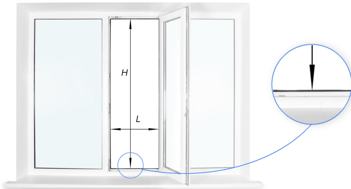
Рис.1. Замер светового проема пластикового окна
